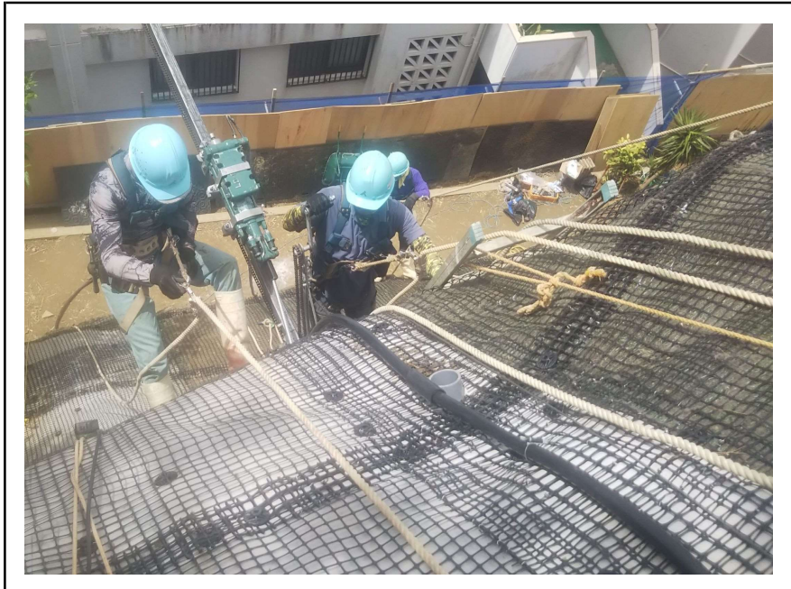
ソイルネイル打設状況
